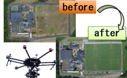
ICT「i-construction」 ドローンを用いた3次元測量
