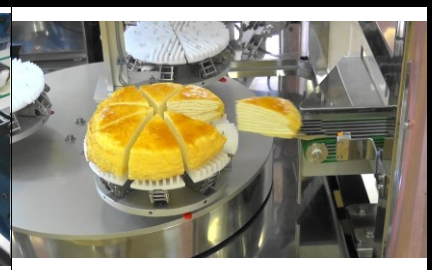
丸ケーキカット装置
